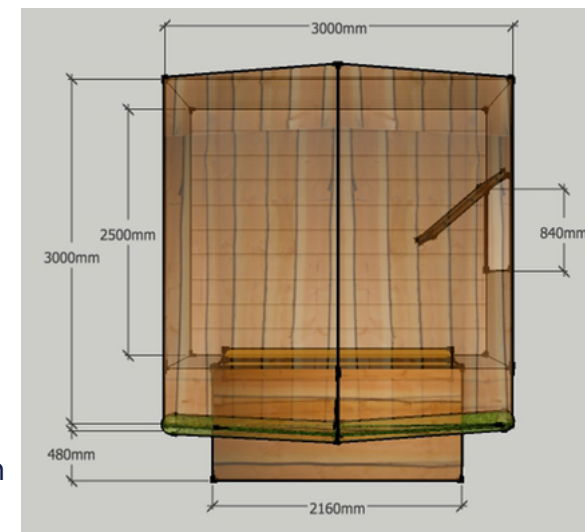
Grondplan chalet:
